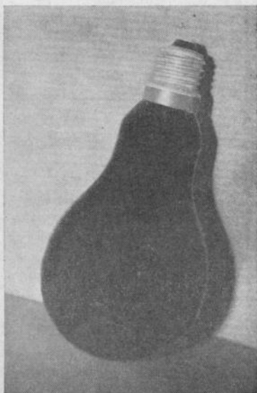
Philips' super hogedruk-kwik-analyselamp Type HPW voor fluorescentie-analyse of luminatie-onderzoek
